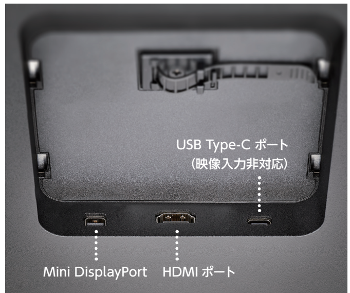
製品背面右側
